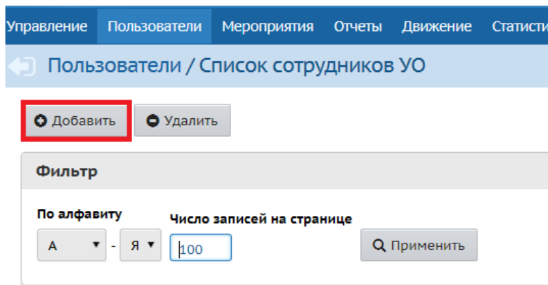
Рис. 5. Добавление пользователя
