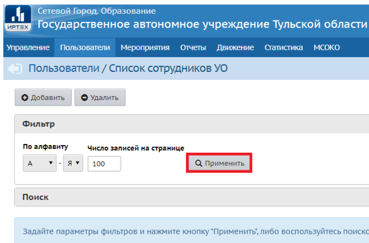
Рис. 2. Просмотр пользователей
